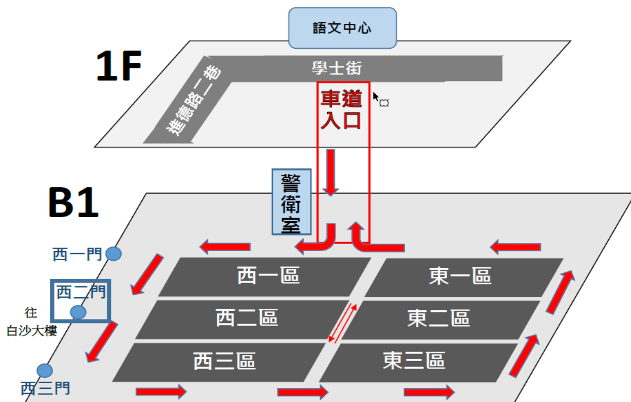
地下室停車場示意圖
